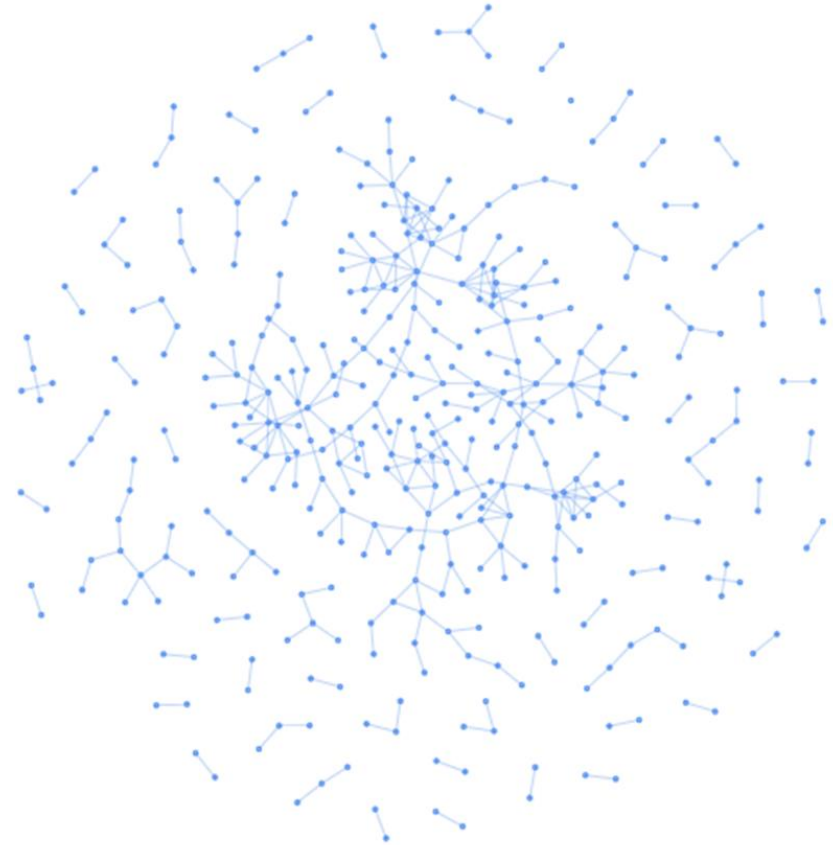
Embedding RDF2Vec
